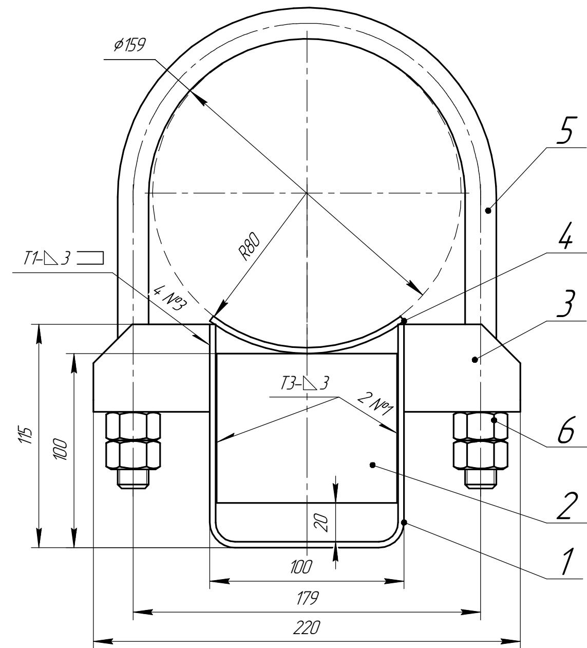
Det. poz. 1
