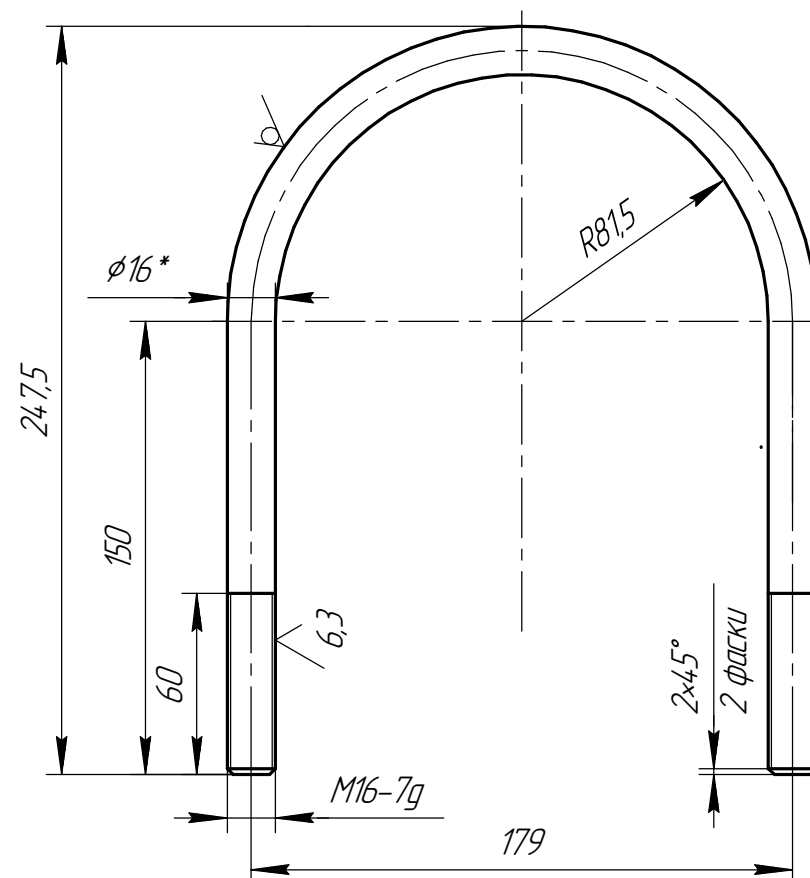
Det. poz. 5 (1:2,5)
