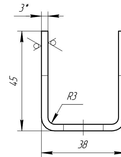
Det. poz. 3 (1:1)
