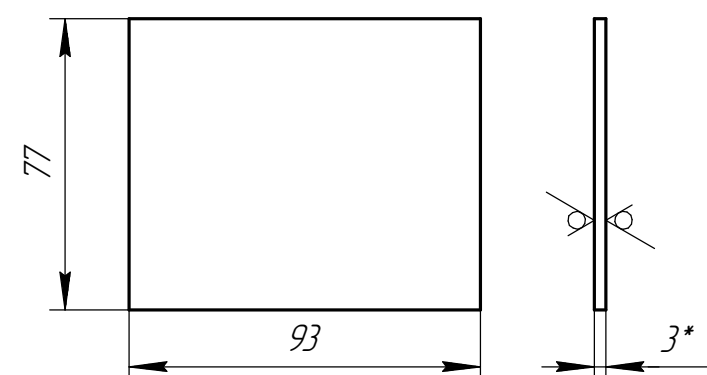
Det. poz. 2
