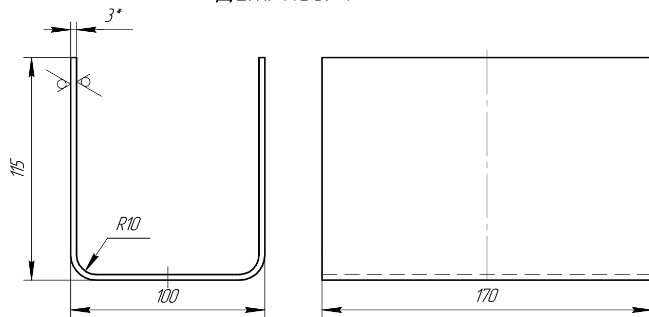
Det. poz. 1
